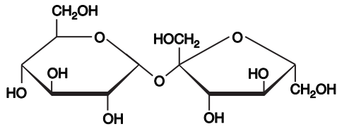
sacharose (bietsuiker/rietsuiker)
